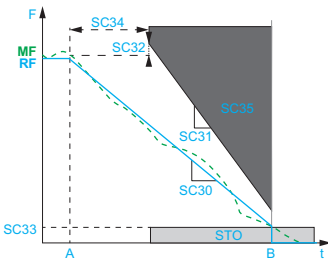
SS1 功能激活
