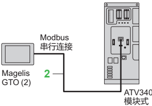
通过Modbus串行连接将模块式ATV340变频器连接至Magelis GTO HMI终端的示例
