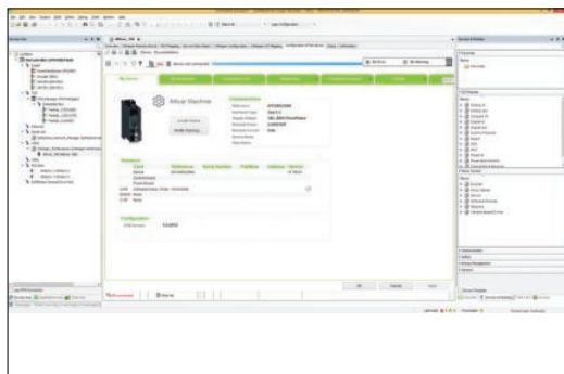
SoMachine中的ATV340DTM
