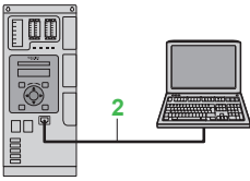
ATV340模块式变频器使用Modbus将变频器与基本中文面板和PC连接
