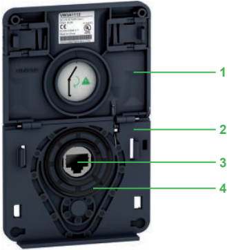
用于在机箱门上安装高级图形终端的远程安装套件(前面)
