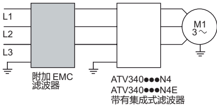
带有附加EMC滤波器的变频器ATV340
