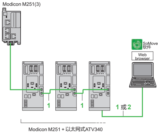
在Ethernet/IP网络上的连接示例
