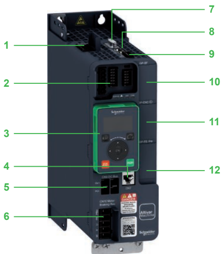
ATV340 以太网式变频器配有基本中文面板
