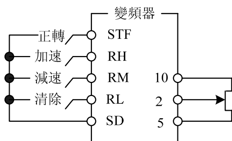
遠端控制設定的接線圖示例
