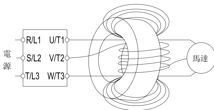
圖 A：將三根輸出線分別在零相電抗器處繞四匝
