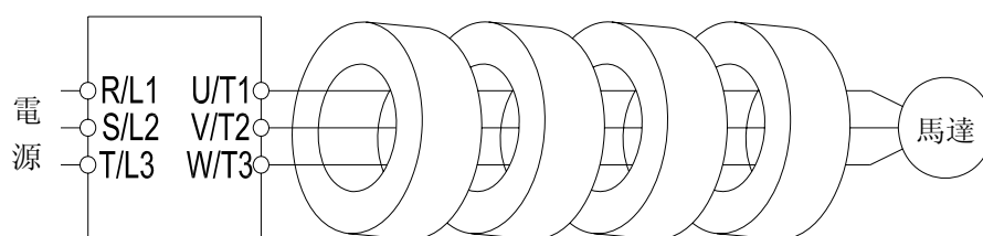
圖 B：將三根輸出線同時穿過四個零相電抗器
