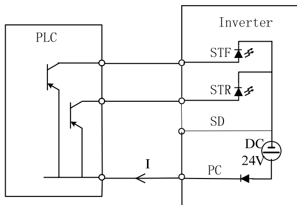
Source Input: 多功能控制端子與開射極的PLC直接連接
